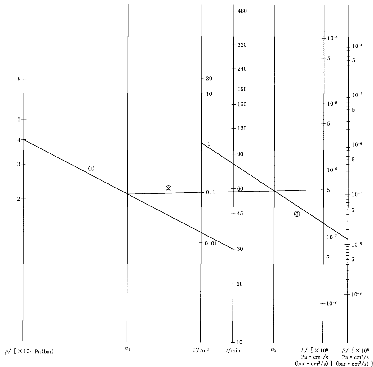
图 D.1 试验参数关系确定
