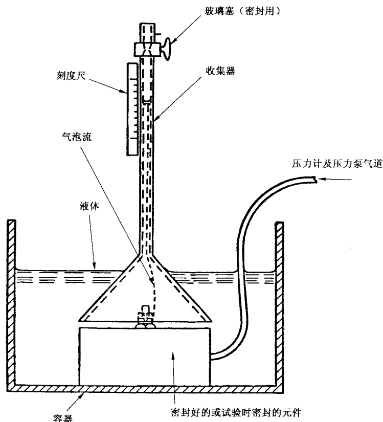
图 A.2 (试验 Qa)密封试验设备
