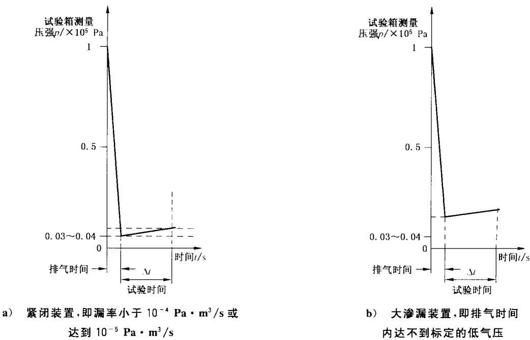
图 4 试验设备规格、测量容积与排气时间为常数的限制条件下,试验箱测量压强与时间的关系
