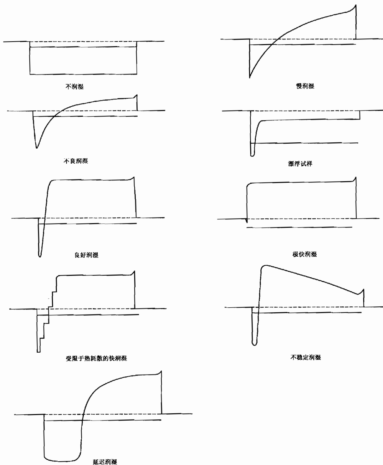
图 B.1 典型的力—时间曲线
