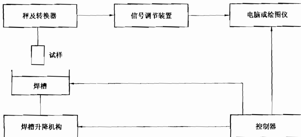
图 1 试验布置图
