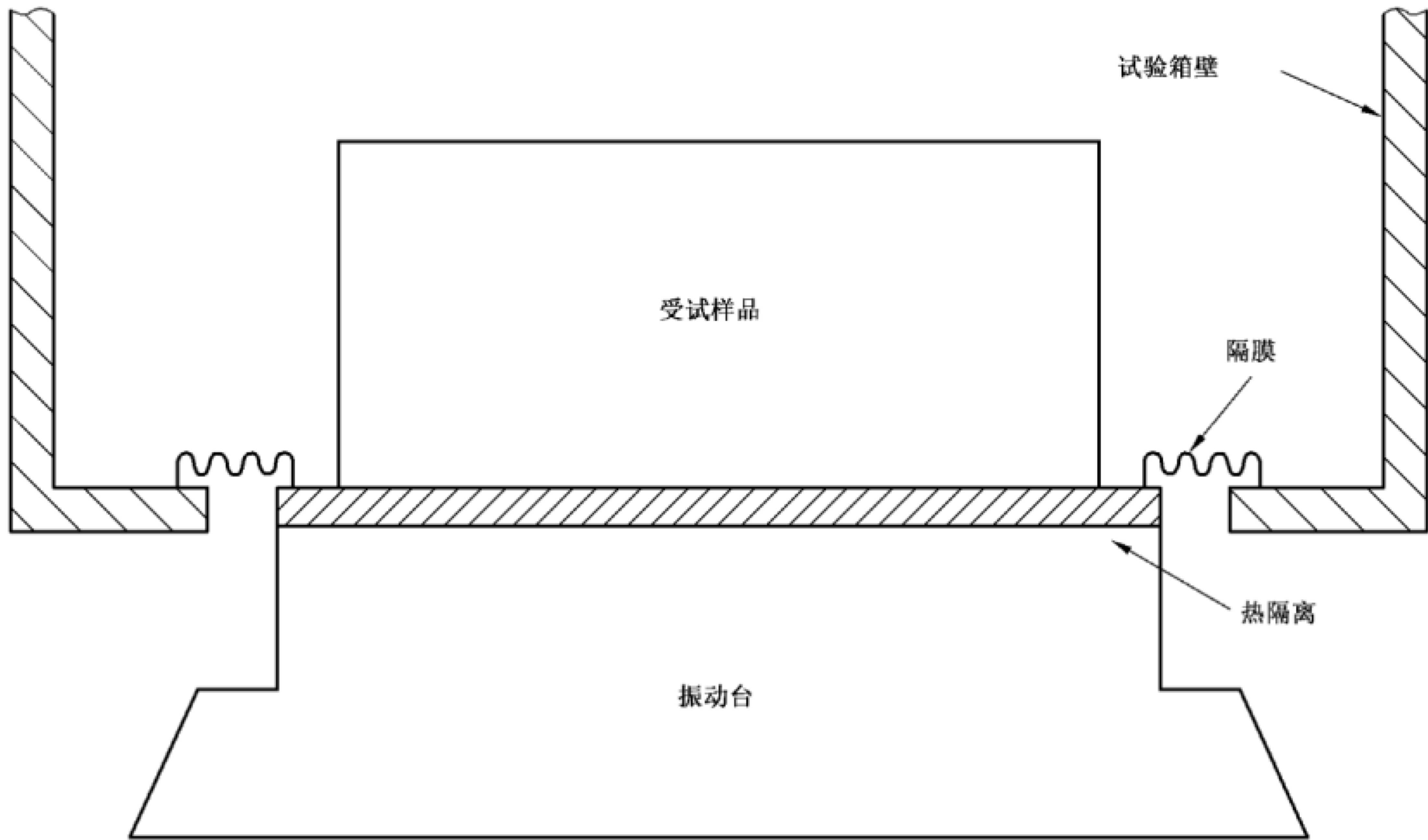
图 B.1 典型试验装置示意
