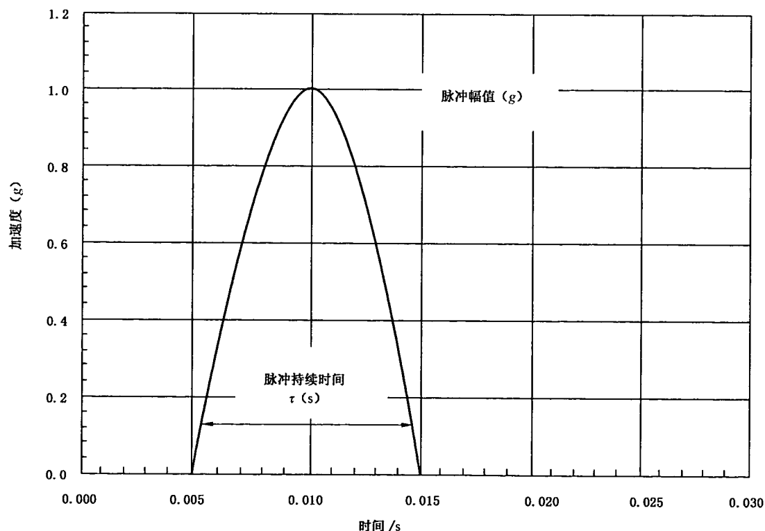
图 C.1 半正弦脉冲的典型特性
