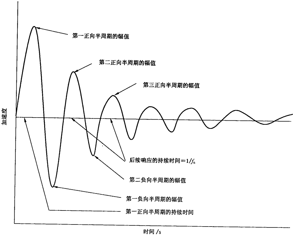
图 C.5 响应特性的记录
