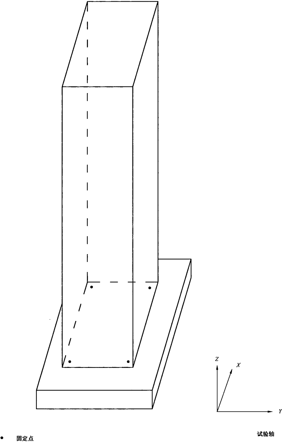
图 5 电子机柜的安装示例
