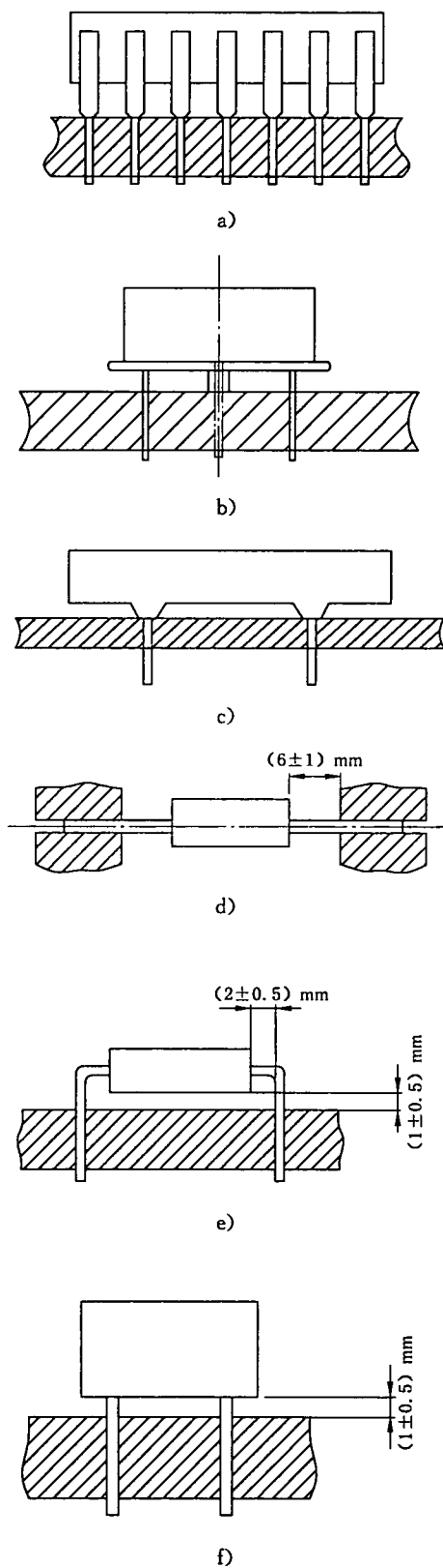
图 2 仅用元件引线安装元件的示例
