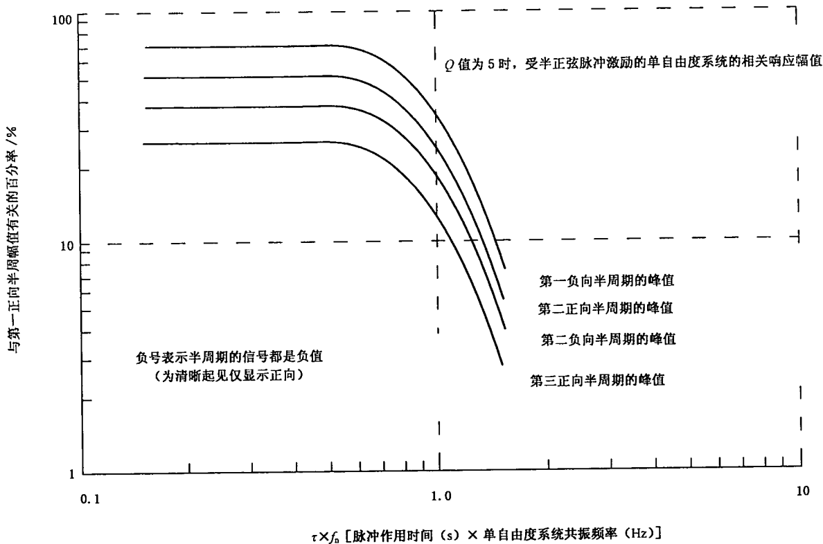
图 C.4 第二响应峰值的相关峰值
