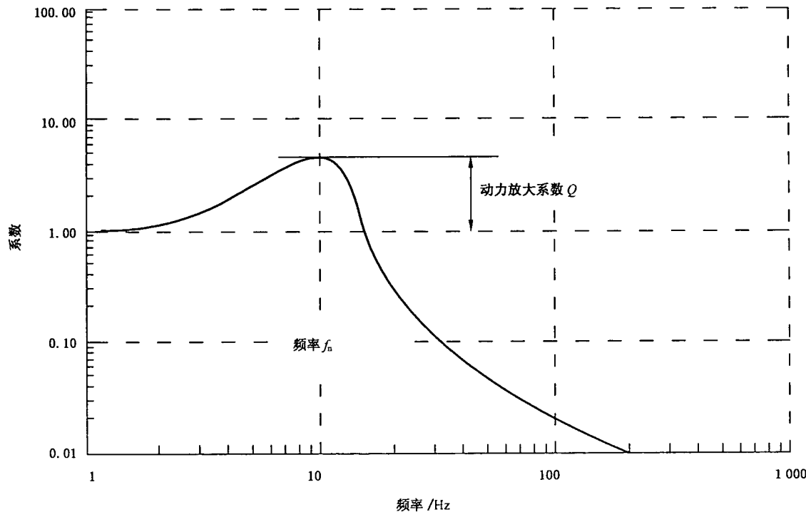
图 C.2 单自由度系统的典型传递特征
